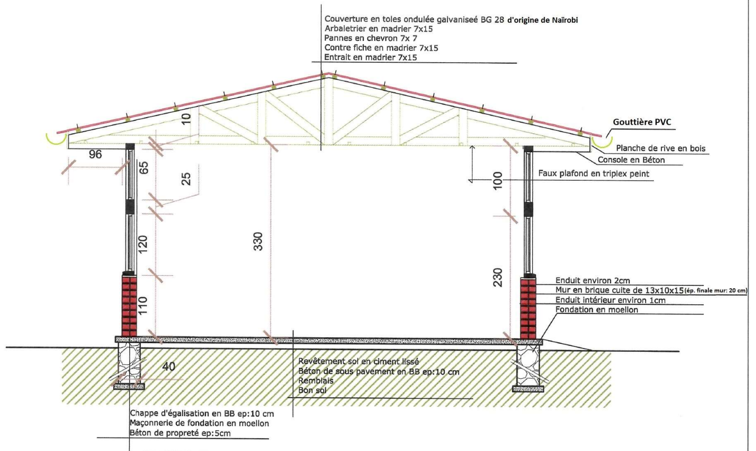
COUPE AA ET PLAN DE LA CHARPENTE
