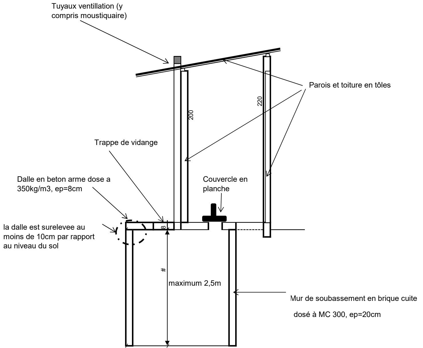
ELEVATION
